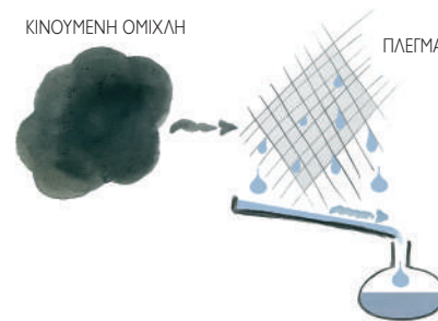
Λειτουργία ομιχλοπαγίδας. Δρόσος, πάχνη και ομίχλη παγιδεύονται σε αναρτημένο πυκνό πλέγμα, συμπυκνώνονται, υγροποιούνται και συλλέγονται με κατάλληλη διάταξη.
