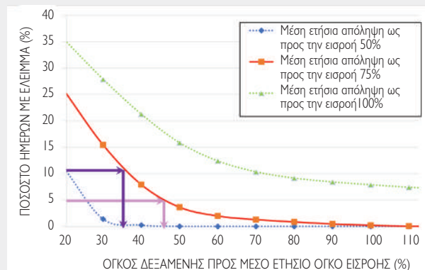
Διάγραμμα 2: Εφαρμογή αδιάστατου διαγράμματος αξιοπιστίας απολήψεων - δεξαμενών ως προς τον ετήσιο όγκο εισροής. Με τα μοβ βέλη μπορεί κάποιος να οδηγηθεί από την αξιοπιστία σχεδιασμού στη διαστασιοποίηση της δεξαμενής.
