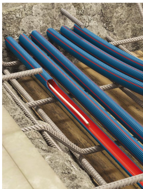
Ο ΣΩΛΗΝΑΣ DUROFLEX® PLUS ΕΙΝΑΙ ΙΔΑΝΙΚΟΣ ΓΙΑ ΤΙΣ ΔΥΣΚΟΛΕΣ ΧΩΝΕΥΤΕΣ ΕΓΚΑΤΑΣΤΑΣΕΙΣ ΣΤΟ ΣΚΥΡΟΔΕΜΑ ΚΑΙ ΕΙΔΙΚΑ ΣΤΗΝ ΟΠΛΙΣΜΕΝΗ ΣΚΥΡΟΔΕΤΗΣΗ ΟΠΟΥ ΑΠΑΙΤΟΥΝΤΑΙ ΥΨΗΛΕΣ ΜΗΧΑΝΙΚΕΣ ΑΝΤΟΧΕΣ.
