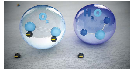
ΤΑ ΑΡΝΗΤΙΚΑ ΦΟΡΤΙΣΜΕΝΑ ΜΟΡΙΑ ΟΞΥΓΟΝΟΥ ΑΝΤΙΔΡΟΥΝ ΜΕ ΤΑ ΜΟΡΙΑ ΥΔΑΤΟΣ ΤΟΥ ΑΕΡΑ.
