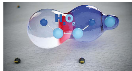
ΑΠΟ ΤΗΝ ΑΝΤΙΔΡΑΣΗ ΤΟΥΣ ΠΡΟΚΥΠΤΕΙ Η 2 O 2 ΚΑΙ ΟΞΥΓΟΝΟ.
