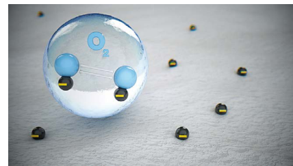
ΤΑ ΜΟΡΙΑ ΟΞΥΓΟΝΟΥ ΤΟΥ ΑΕΡΑ (O 2 ) ΠΡΟΣΛΑΜΒΑΝΟΥΝ ΤΑ ΑΡΝΗΤΙΚΑ ΦΟΡΤΙΣΜΕΝΑ ΗΛΕΚΤΡΟΝΙΑ.
