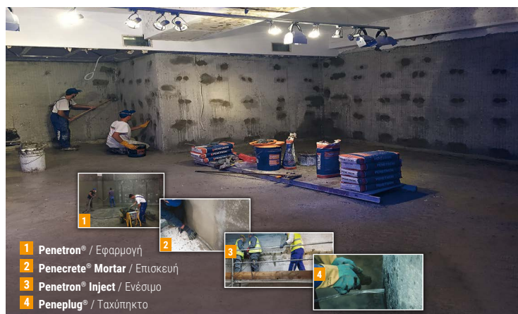
ΒΗΜΑ 3: ΕΠΙΣΚΕΥΗ ΜΟΡΕΛΩΝ, ΦΩΛΕΩΝ ΚΑΙ ΑΔΟΝΗΤΩΝ ΣΤΟ ΣΚΥΡΟΔΕΜΑ ΜΕ ΣΥΜΒΑΤΑ ΚΟΝΙΑΜΑΤΑ ΤΟΥ ΣΥΣΤΗΜΑΤΟΣ PENETRON® ΜΕ ΑΝΑΠΤΥΞΗ ΚΡΥΣΤΑΛΛΩΝ.
